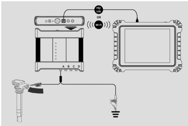
図7 -1 接続図
