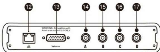
図2 -7 VCM1底面図
