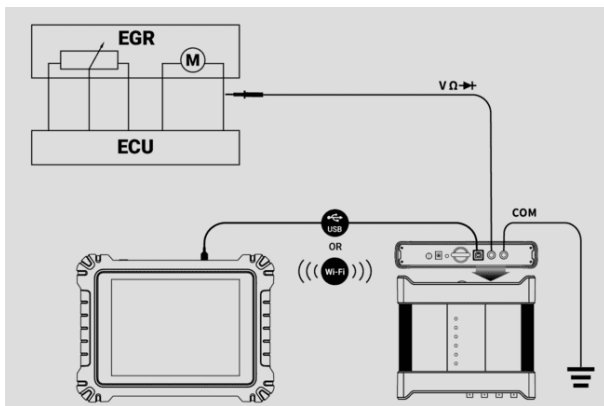
図7 -93 アクチュエーター駆動接続図
