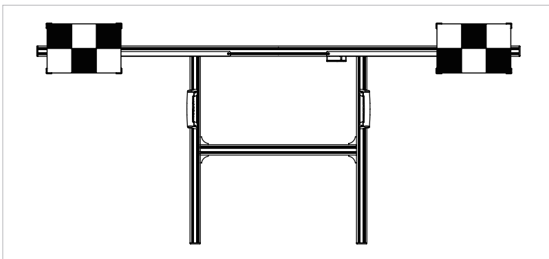
SOPORTE DE TABLERO DE OBJETIVOS LDWII 0600-22
